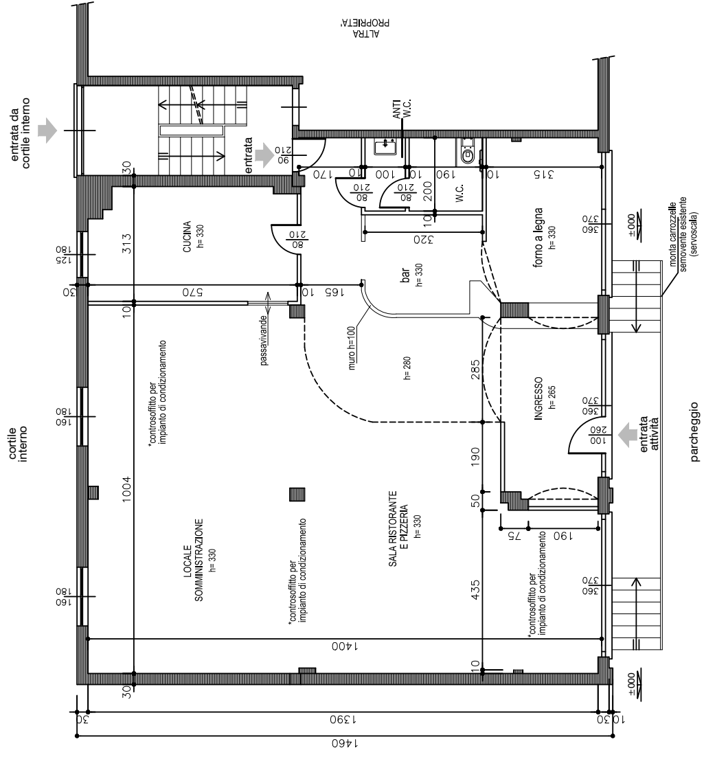
disegno 1 Pianta Piano Rialzato Stato di Fatto 1:100
